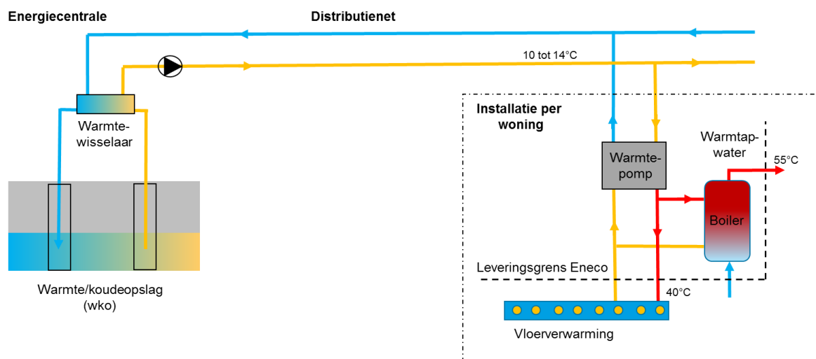
figuur 2.1 Het wko-systeem
