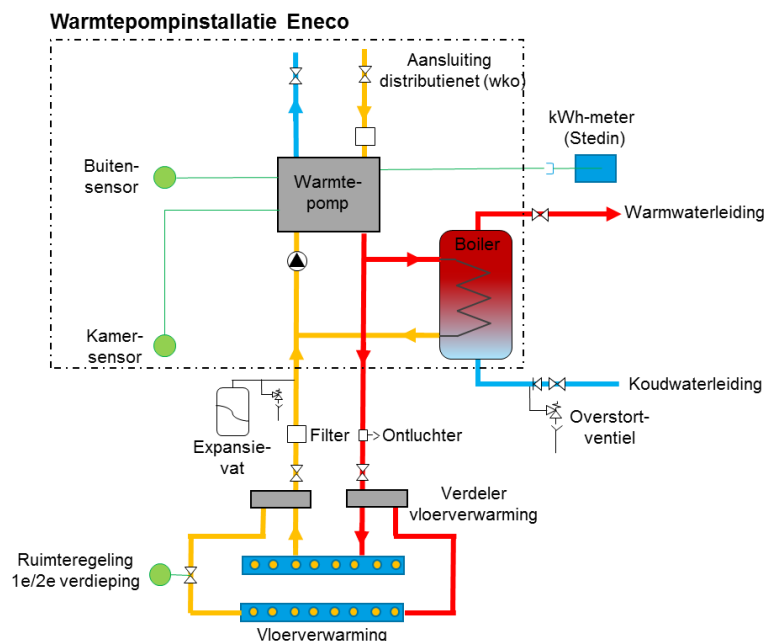
figuur 2.2 De warmtepompinstallatie in de woningen
