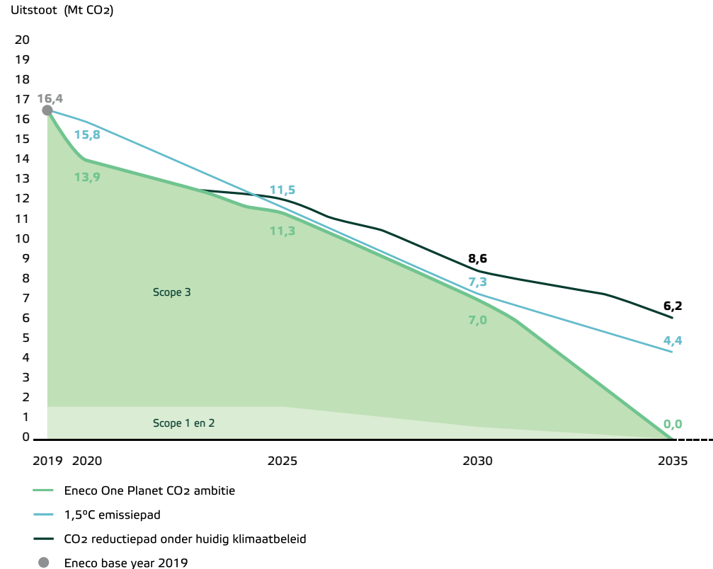
Figuur 11: Huidig beleid is niet toereikend om onder het 1,5°C-pad te blijven
