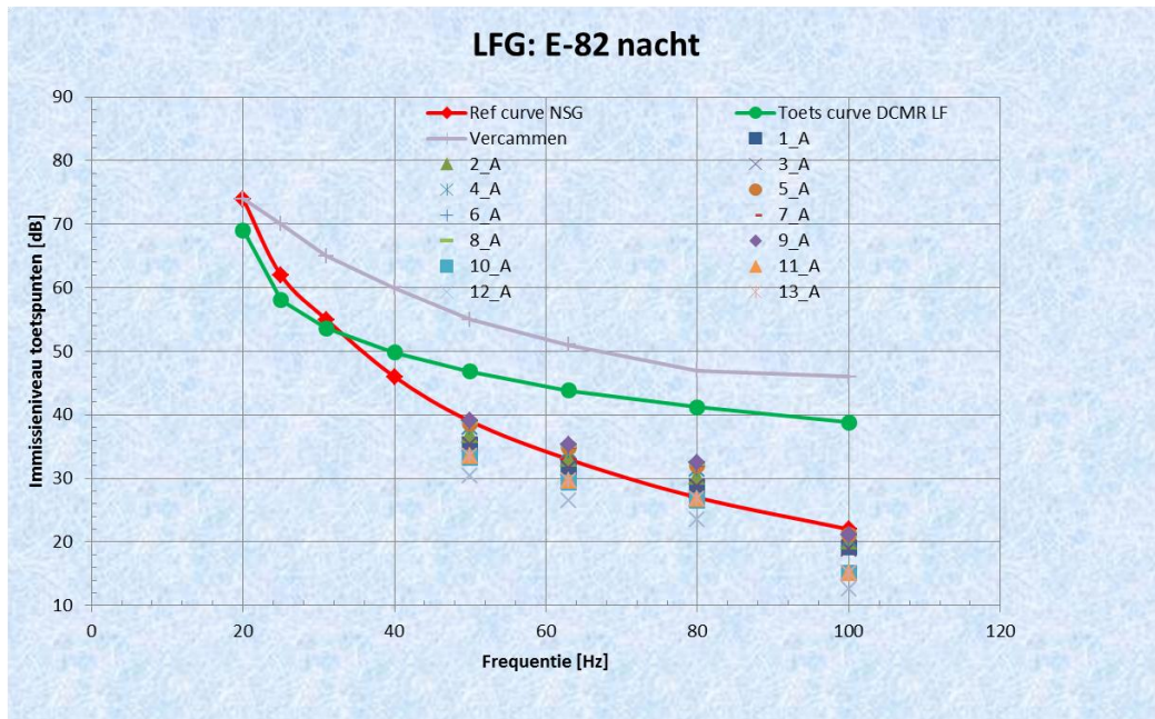
Grafiek 1: laagfrequent geluid 9x Enercon E-82 E2 2,3 MW nacht.
