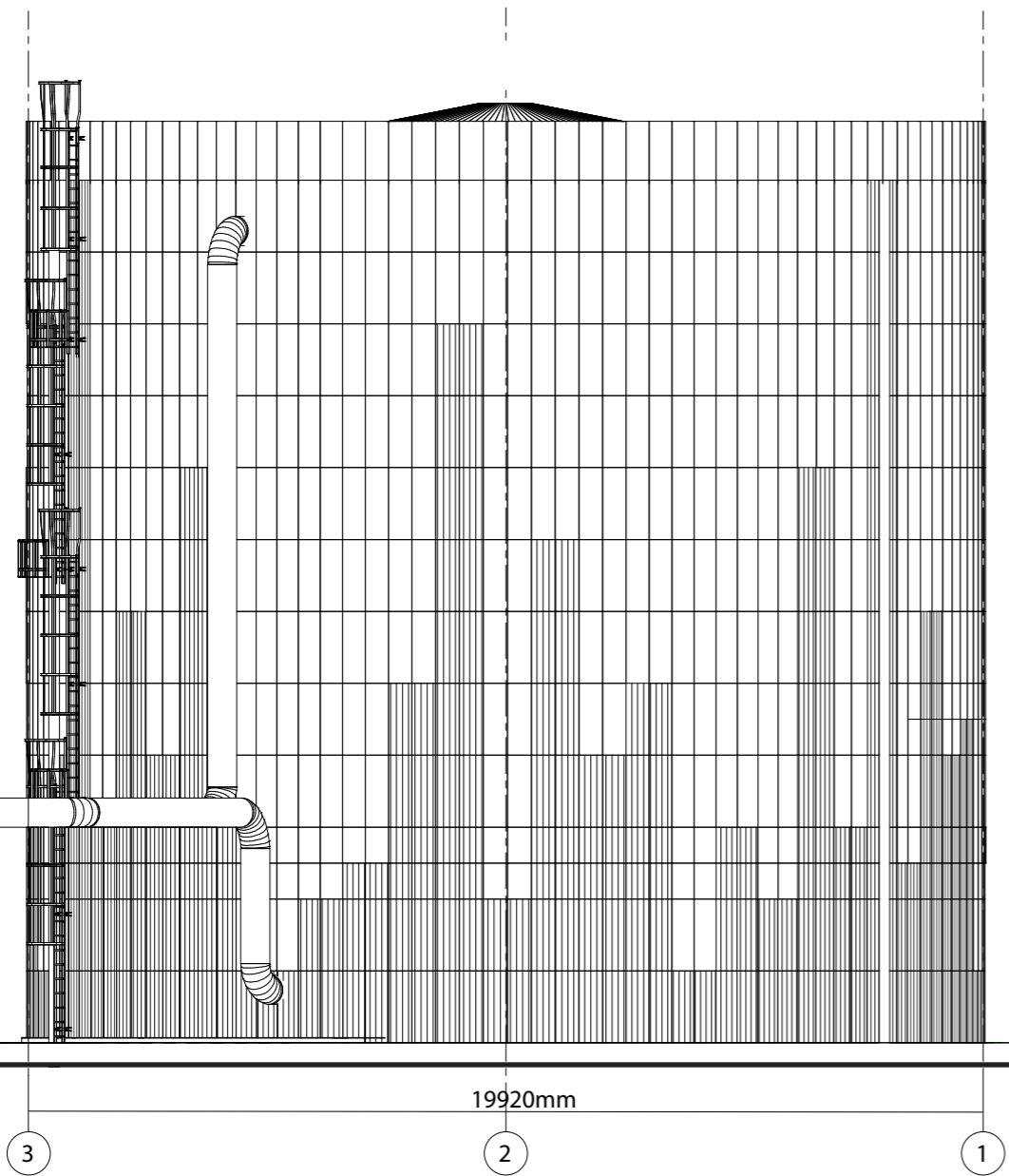
Noordgevel
