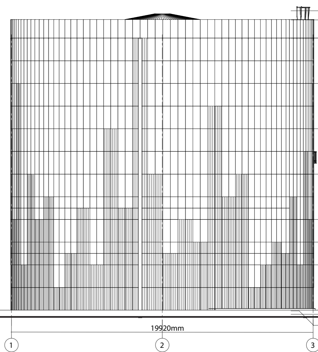
Zuidgevel
